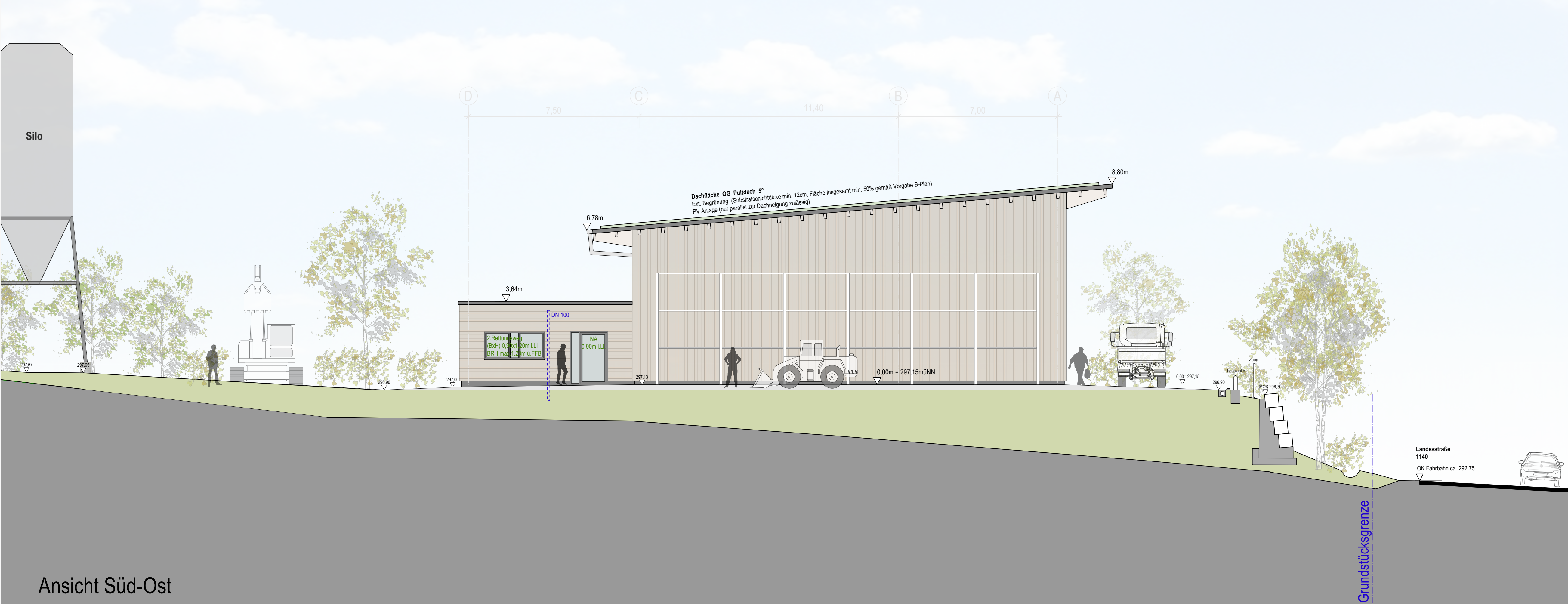
Ansicht Süd-West
