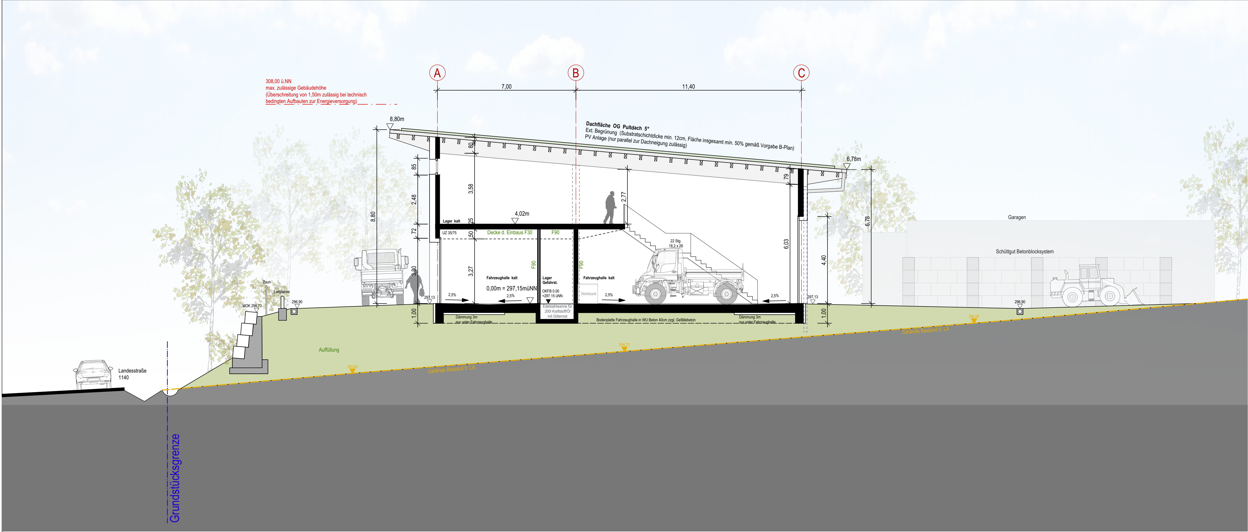
Schnitt A-A
