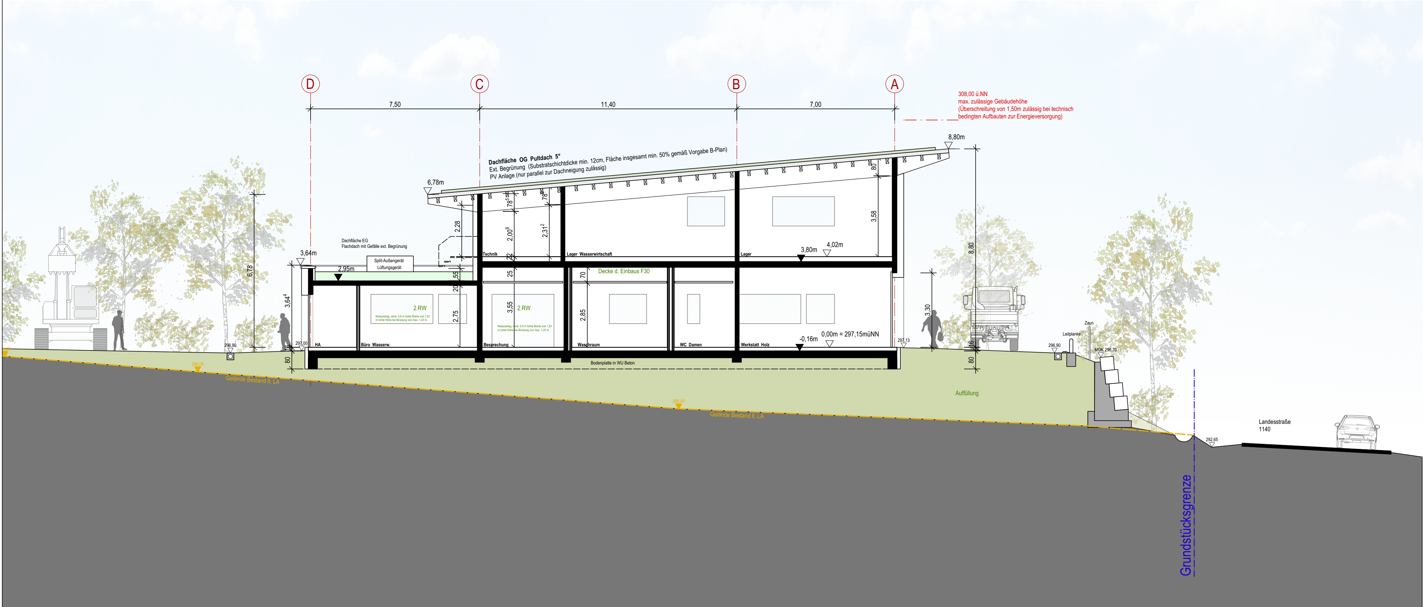
Schnitt B-B
